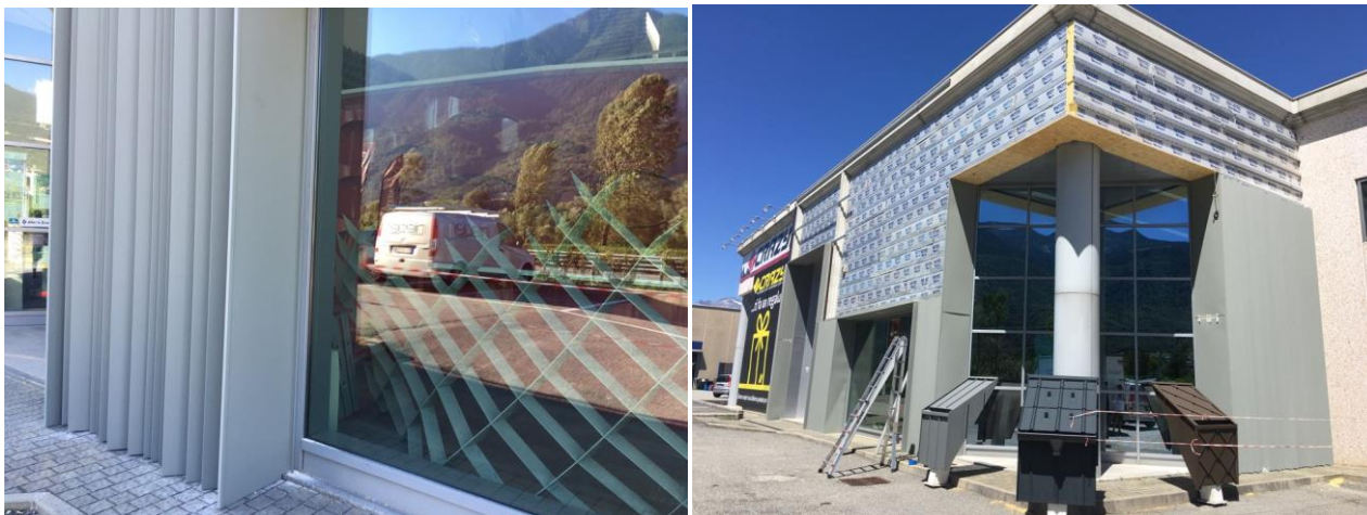
Le fasi della posa di ISOTEC PARETE sull'edificio esistente e del rivestimento metallico sulla facciata.
